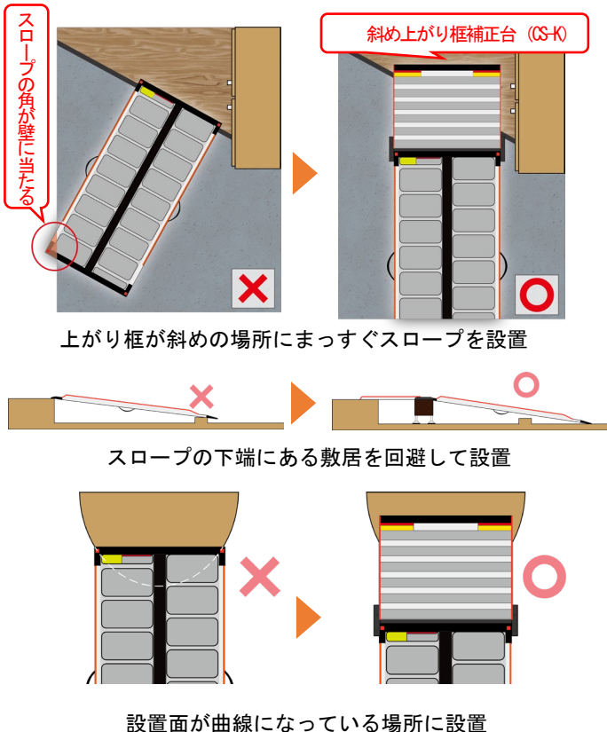
▲専用斜め上がり框補正台
